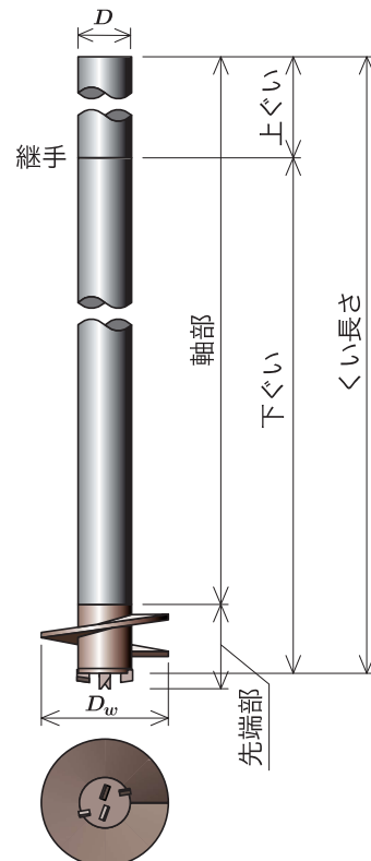
各部名称
